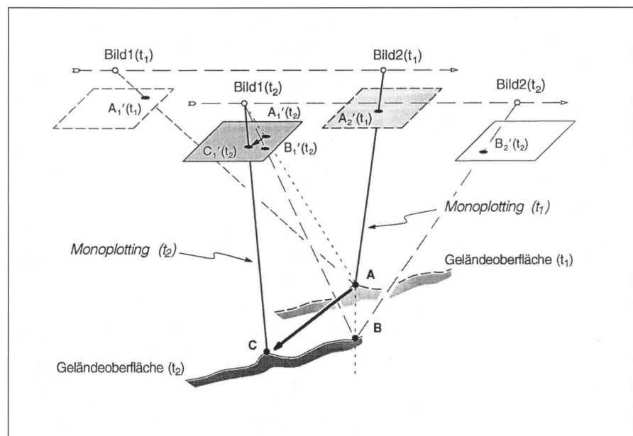
Abb. 6: Mono- und multitemporale Stereomodelle und Bewegungsmessung durch simultanes Monoplething.
