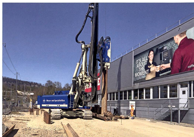
Einbau Rühlwände (März 2021).
