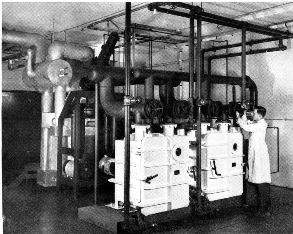
Ansicht einer modernen Dehydrierungs-Anlage und schematische Darstellung einer solchen Einrichtung. Die durch uns installierte Blut-Dehydrierungs-Anlage für das Schweizerische Rote Kreuz umfasst ebenfalls diese Hauptbestandteile.
