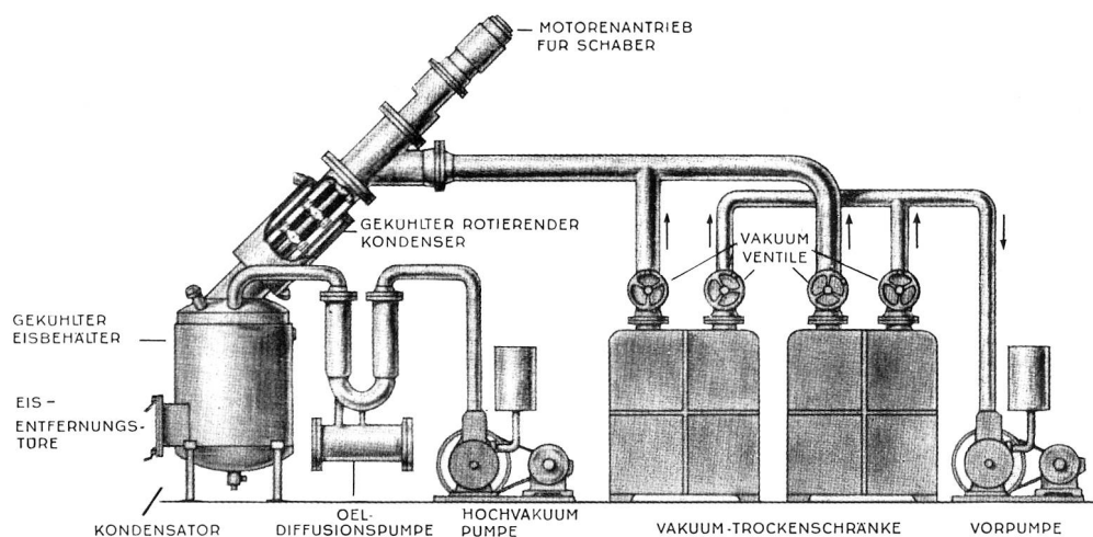
Ansicht einer modernen Dehydrierungs-Anlage und schematische Darstellung einer solchen Einrichtung. Die durch uns installierte Blut-Dehydrierungs-Anlage für das Schweizerische Rote Kreuz umfasst ebenfalls diese Hauptbestandteile.
