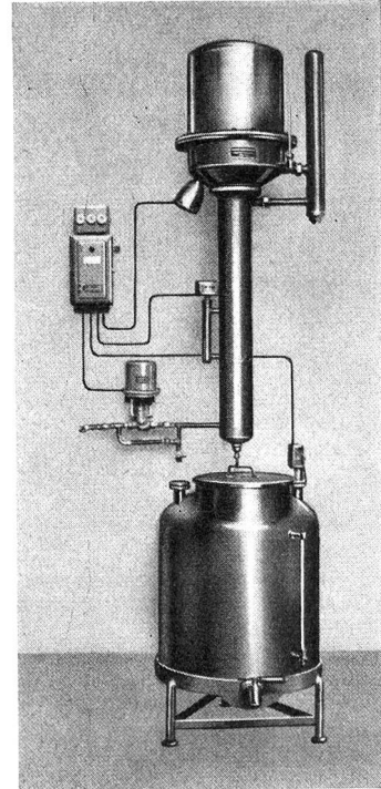
Elektrisch beheizter UNITYP KBC mit Reservoir in Kupfer oder Steinzeug
