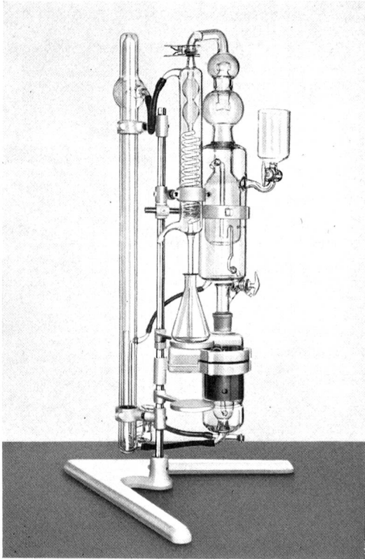
Apparat zur Stickstoffbestimmung
