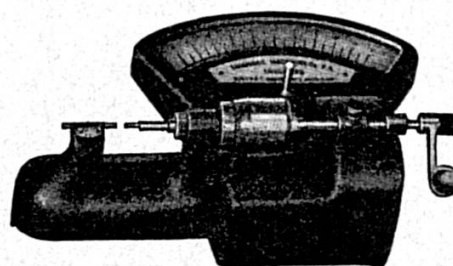
MICROMÈTRE- COMPARATEUR
