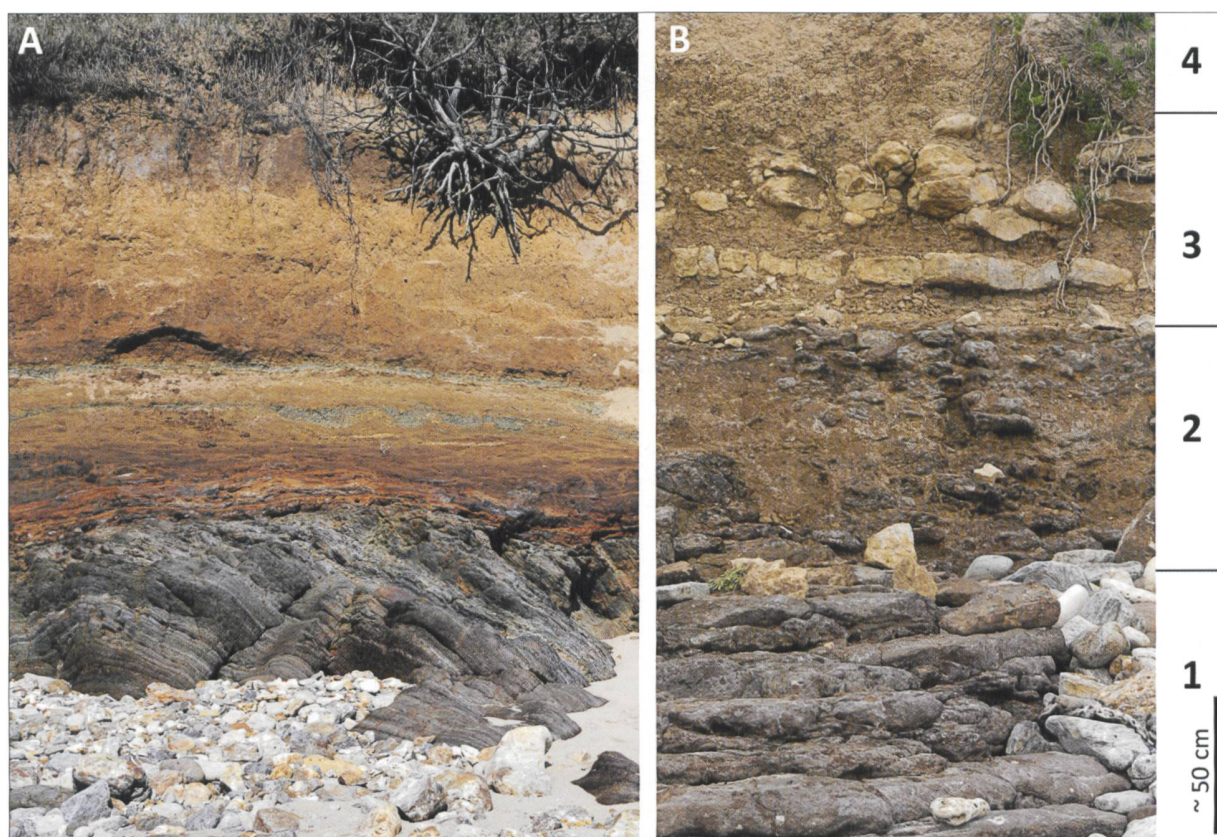
Fig. 2. A) Discontinuité angulaire du Jurassique basal sur les schistes et gneiss. Pointe du Payré à proximité du chemin de la ferme de St-Nicolas; B) Coupe du gisement de St-Nicolas. 1. couches dolomitiques du Sinémurien ou de l'Hettangien, 2. calcaires bruns et marnes vertes du Sinémurien ou de l'Hettangien (les gastéropodes et les algues ont été récoltés dans les 20 derniers centimètres), 3. calcaires et marnes beiges du Pleinsbachien (Carixien), 4. dépôts dunaires quaternaires.
