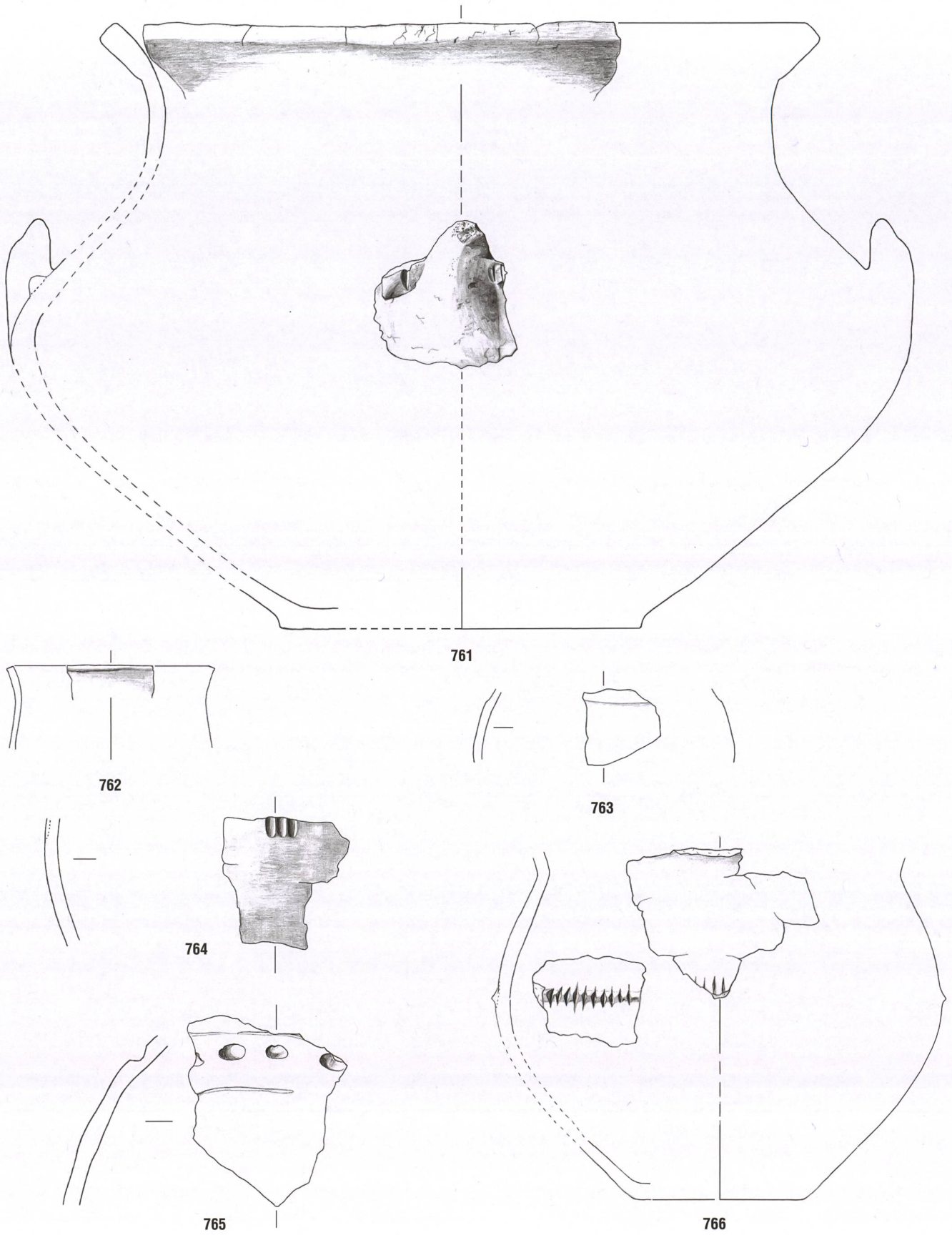
Tafel 58: Cazis, Cresta 1947-1970. Südliche Zentralspalte, Keramikhorizont KH III. 761-766: Planum 9S. Keramik. Mst. 1:3.
