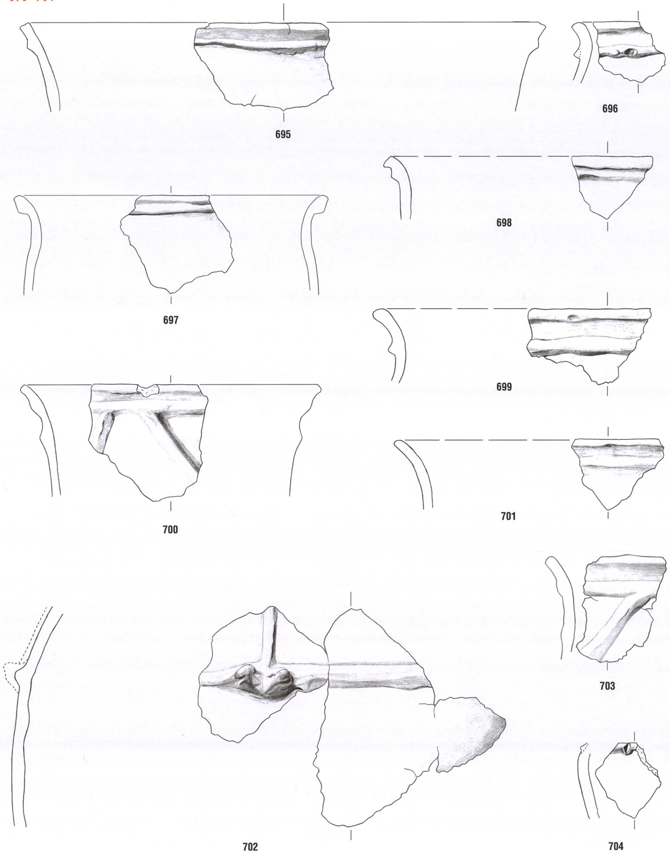
Tafel 52: Cazis, Cresta 1947-1970. Südliche Zentralspalte, Keramikhorizont KH II. 695-704: Planum 6S. Keramik. Mst. 1:3.
