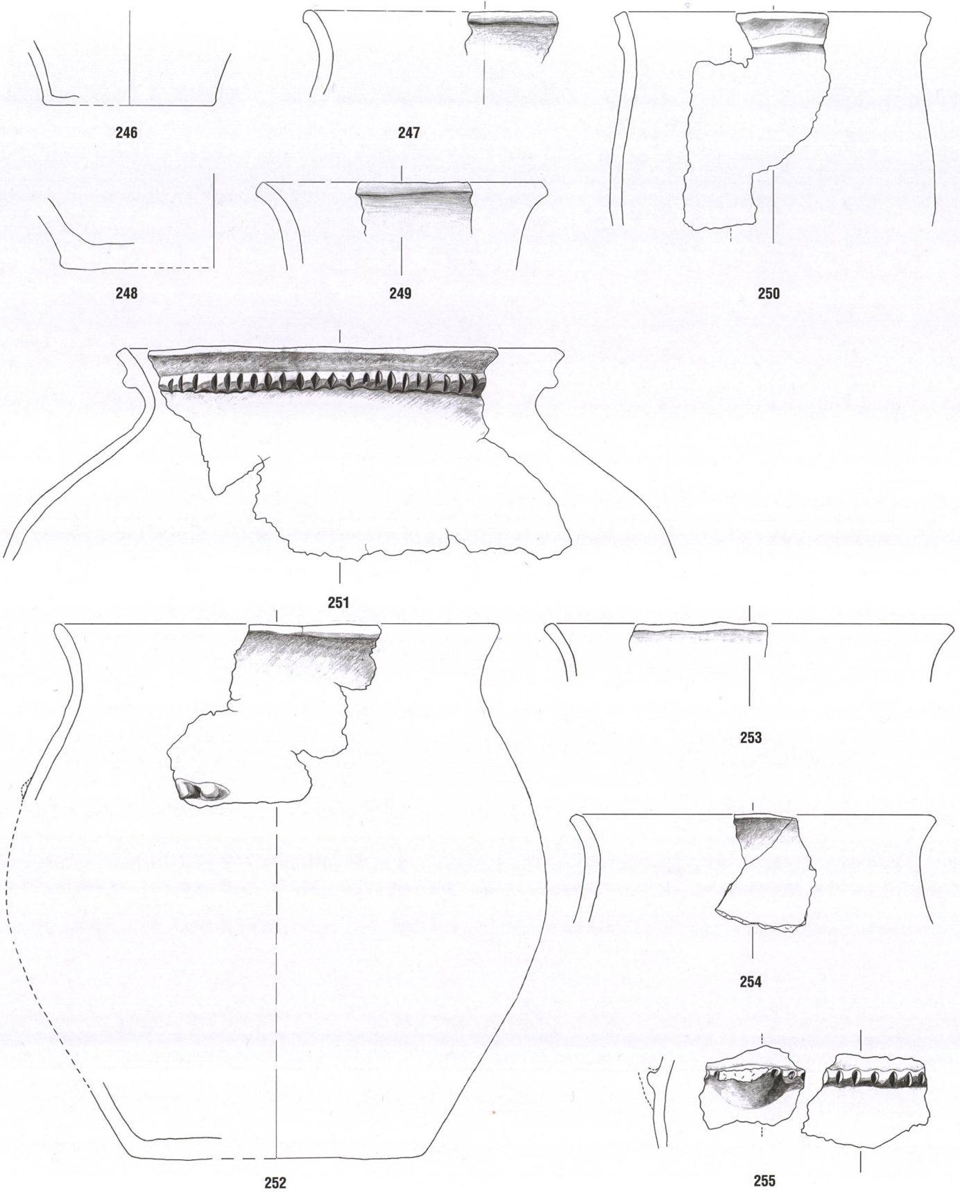
Tafel 20: Cazis, Cresta 1947–1970. Nördliche Zentralspalte, Keramikhorizont KH II. 246–247: Planum 7N oder 8N. 248–249: Planum 7N. 250–254: Planum 8 N. 255: Planum 6N. Keramik. Mst. 1:3.
