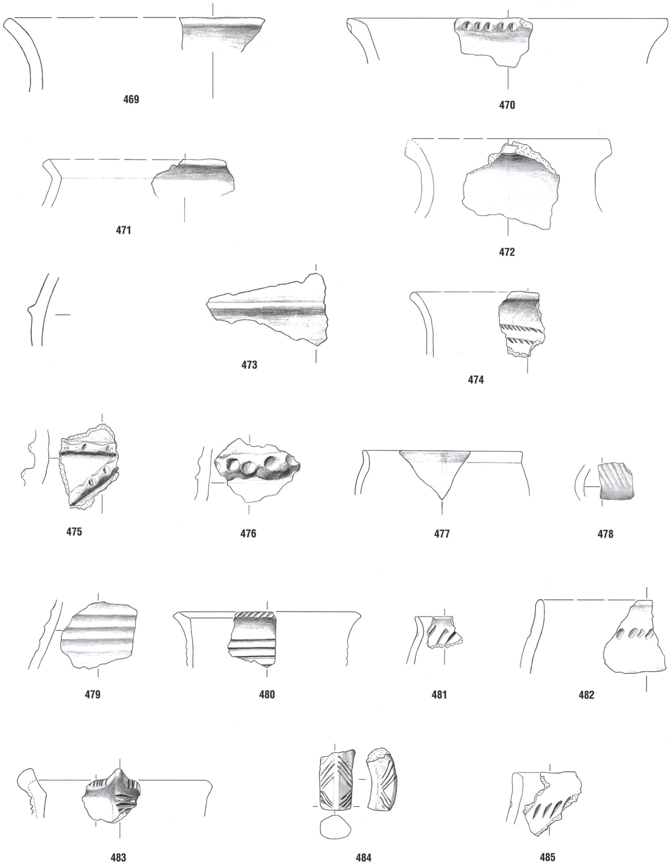
Tafel 39: Cazis, Cresta 1947–1970. Nördliche Zentralspalte, Keramikhorizont KH IV. Aus dem gestörten Bereich der Felder 17 und 18. 469–470: Planum 9N. 471–481: Planum 10N. 483–484: Plana 10N–11N. 482, 485: Planum 11N. Keramik. Mst. 1:3.
