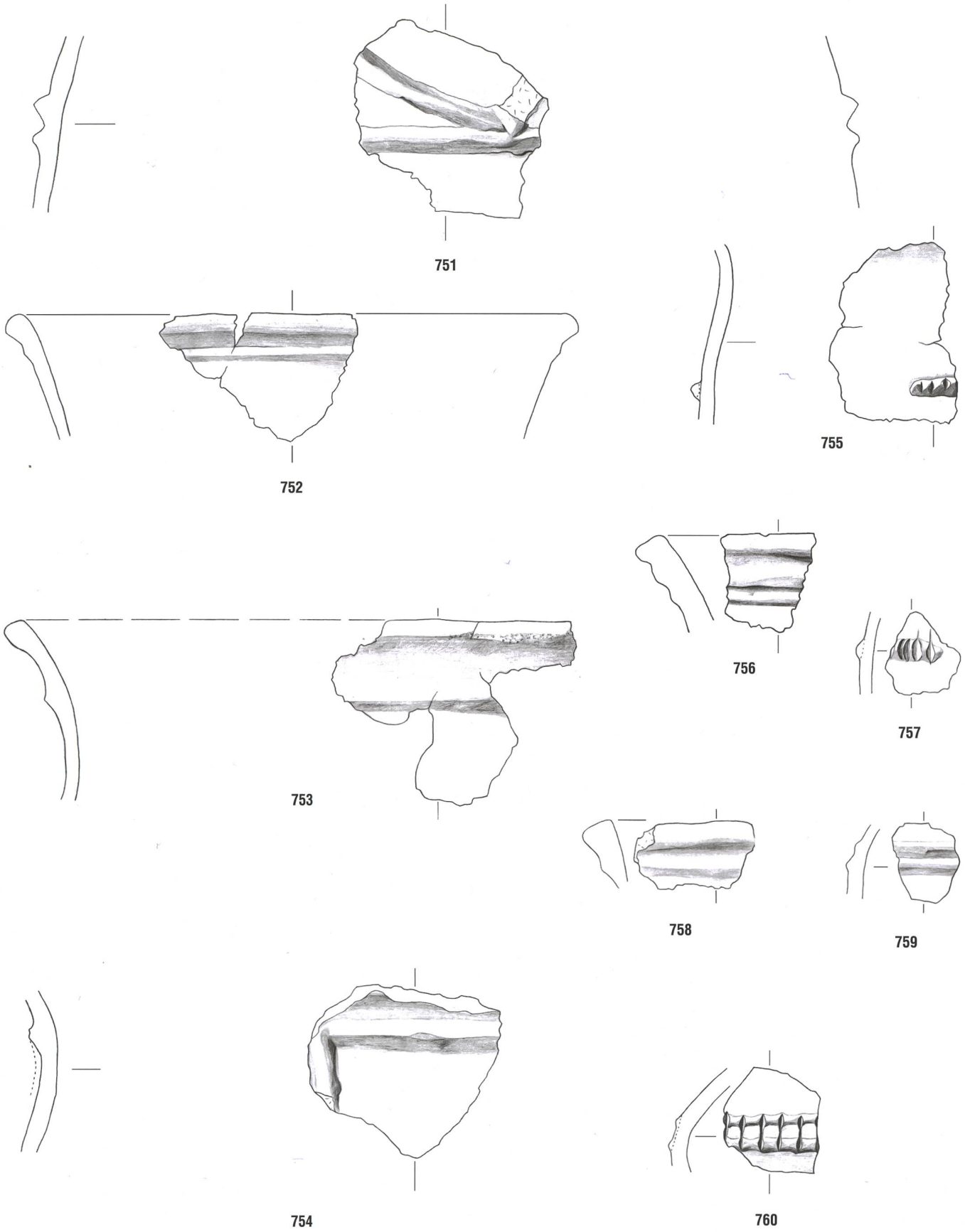
Tafel 57: Cazis, Cresta 1947-1970. Südliche Zentralspalte, Keramikhorizont KH III. 751-760: Planum 9S. Keramik. Mst. 1:3.
