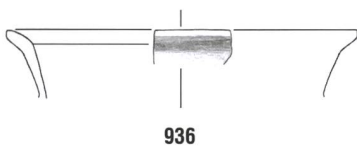
Tafel 73: Cazis, Cresta 1947-1970. Südliche Zentralspalte, Keramikhorizont KH IV. 921-940: Planum 12S. Keramik. Mst. 1:3.
