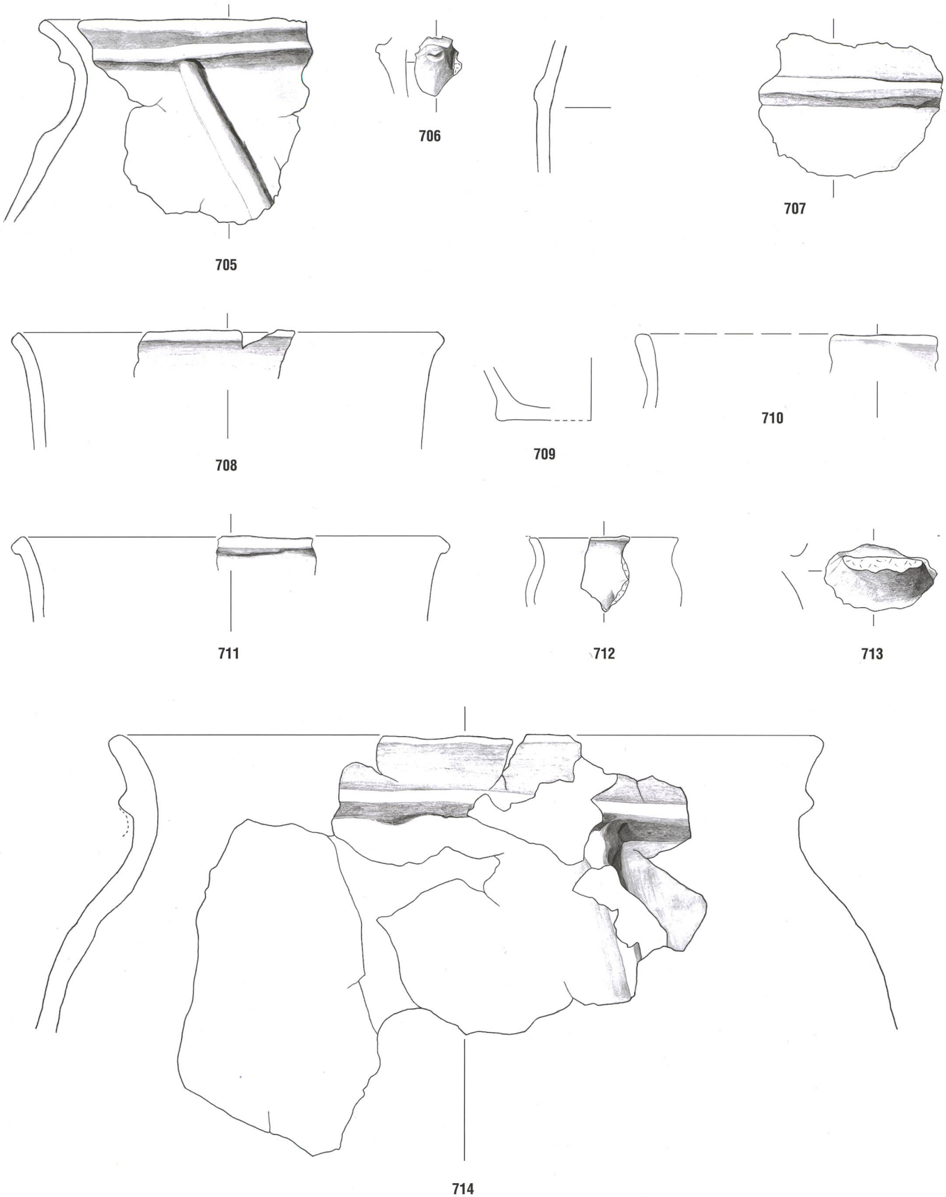
Tafel 53: Cazis, Cresta 1947-1970. Südliche Zentralspalte, Keramikhorizont KH II. 705-713: Planum 6S. 714: Planum 7S. Keramik. Mst. 1:3.
