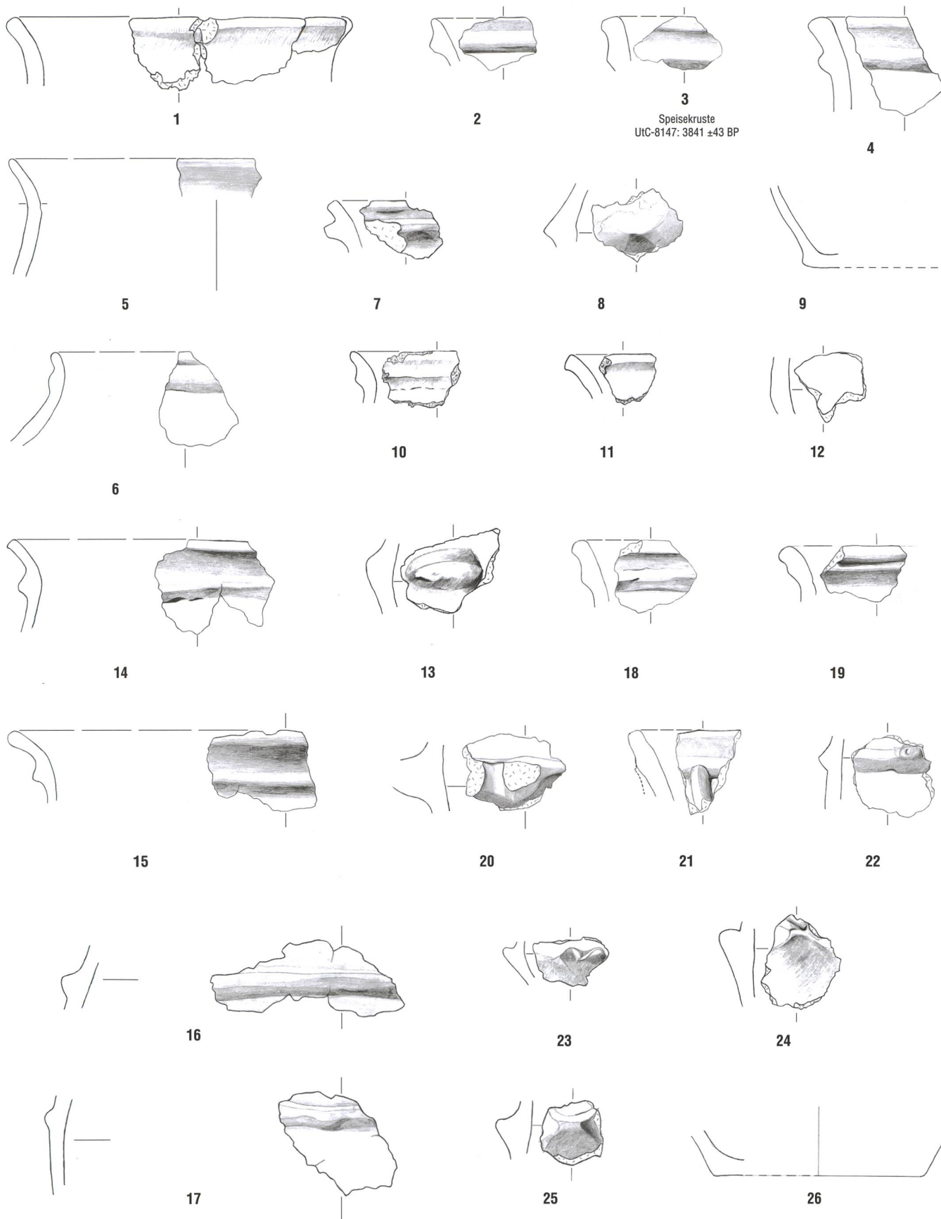
Tafel 1: Cazis, Cresta 1947–1970. Nördliche Zentralspalte, Keramikhorizont KH I. 1–9: Planum 1N. 10–13: zwischen Planum 1aN und 3aN. 13–26: Planum 2N. Keramik. Mst. 1:3.
