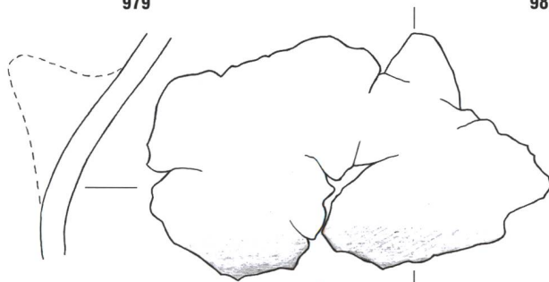
Tafel 75: Cazis, Cresta 1947-1970. Südliche Zentralspalte, Keramikhorizont KH IV. 966-983: Planum 12S. Keramik. Mst. 1:3.
