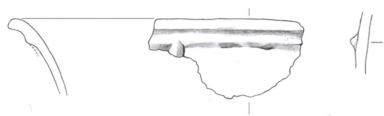
Tafel 33: Cazis, Cresta 1947-1970. Nördliche Zentralspalte, Keramikhorizont KH III. 382-391: Planum 12N. Keramik. Mst. 1:3.
