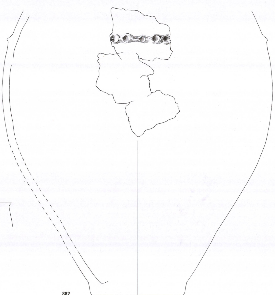
Tafel 70: Cazis, Cresta 1947-1970. Südliche Zentralspalte, Keramikhorizont KH III. 876-882: Planum 9S. Keramik. Mst. 1:3.
