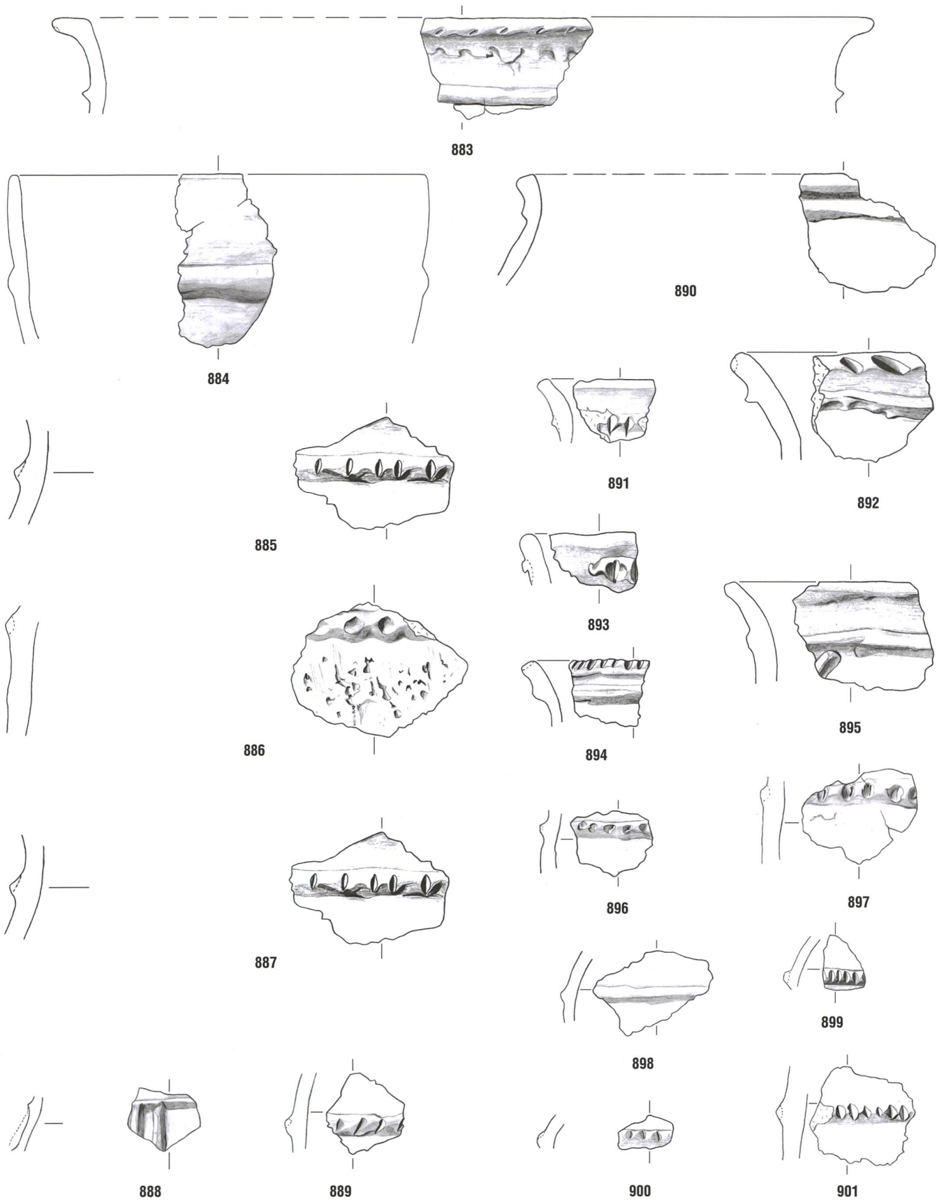
Tafel 71: Cazis, Cresta 1947-1970. Südliche Zentralspalte, Keramikhorizont KH IV. 883-901: Planum 12S. Keramik. Mst. 1:3.
