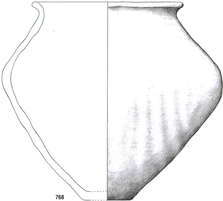
Tafel 59: Cazis, Cresta 1947-1970. Südliche Zentralspalte, Keramikhorizont KH III. 767-775: Planum 9S. Keramik. Mst. 1:3.
