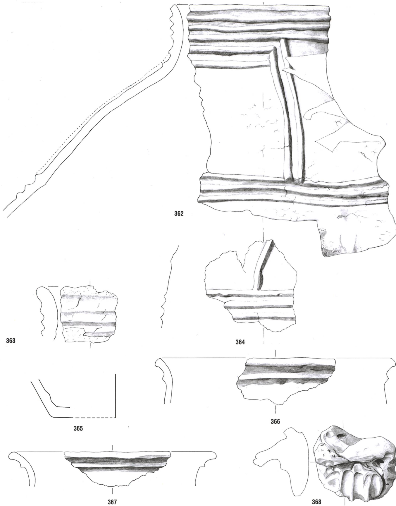
Tafel 31: Cazis, Cresta 1947–1970. Nördliche Zentralspalte, Keramikhorizont KH III. 362–368: Planum 12N. Keramik. Mst. 1:3.
