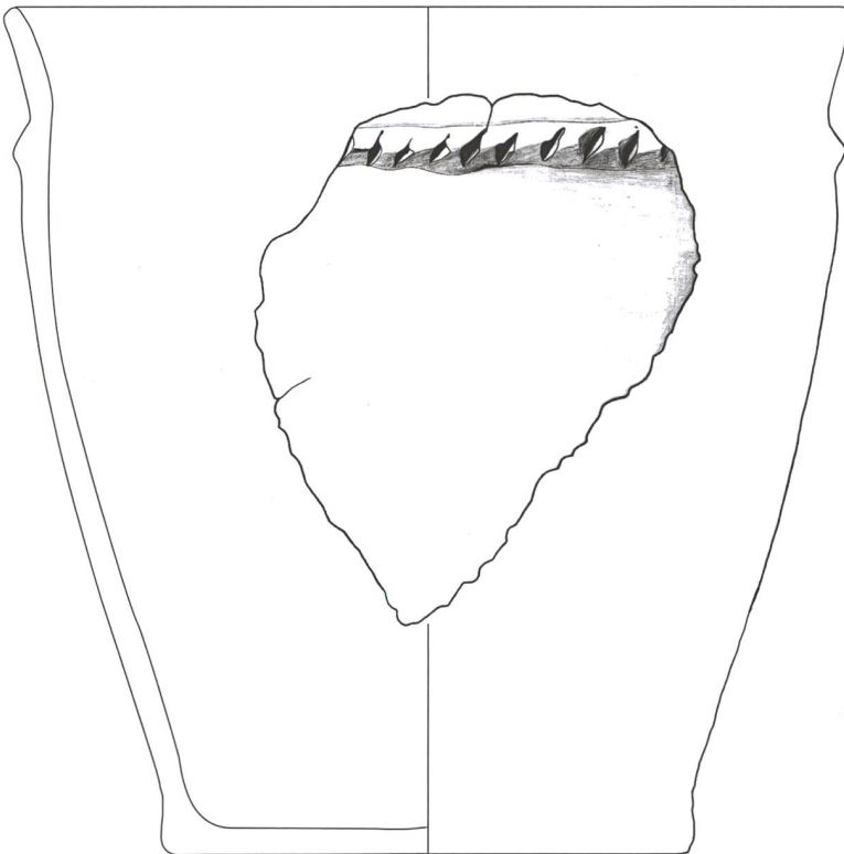
Tafel 91: Cazis, Cresta 1947–1970. 1225–1228: Nordspalte. 1229–1231: Ostfelder. 1232, 1233: Streufunde. Keramik. Mst. 1:3.
