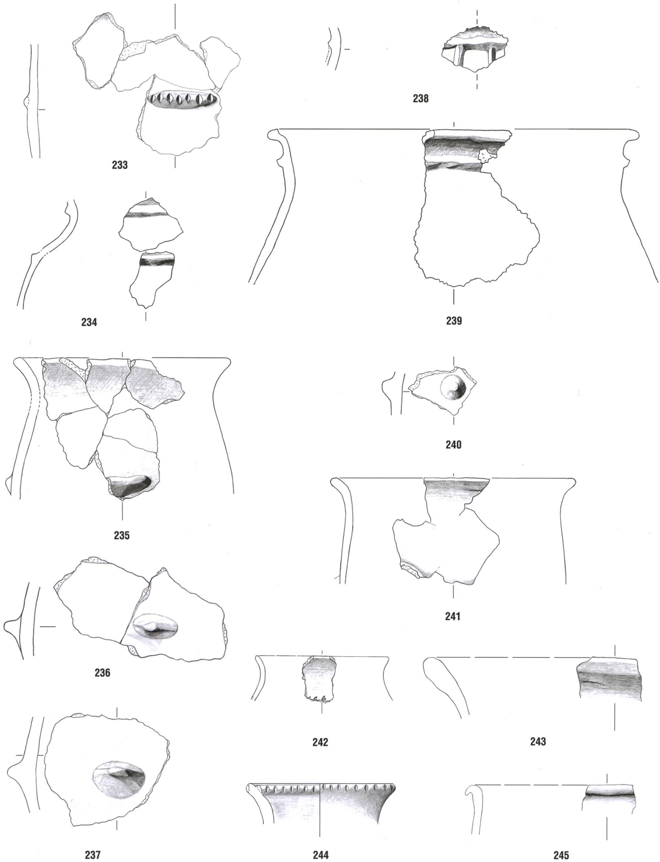
Tafel 19: Cazis, Cresta 1947–1970. Nördliche Zentralspalte, Keramikhorizont KH II. 233–235, 240–241, 243, 245: Planum 7N oder 8N. 236–237, 242, 244: Planum 7N. 238–239: Planum 8N. Keramik. Mst. 1:3.
