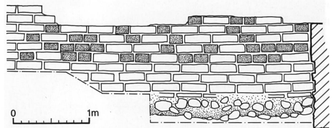
Abb.16: Mauertechnik der Backsteinmauer. Dunkel gepunktet die Bindelagen, weiss die Läufer. M. 1:50.
