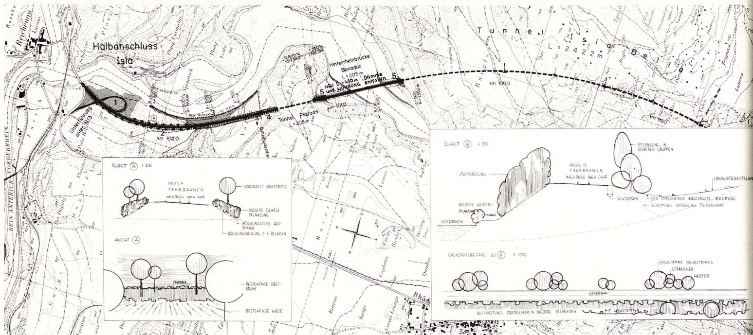
Ausschnitt aus dem Gestaltungsplan der Diplomarbeit F. Schutz, 1976. «Studie zur Eingliederung der N 13 im Raume Thuisis».
