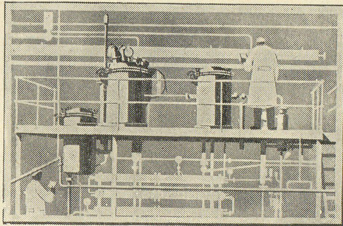
Die neuartige Uperisations-Anlage in der Ovomaltine-Fabrik Neuenegg
