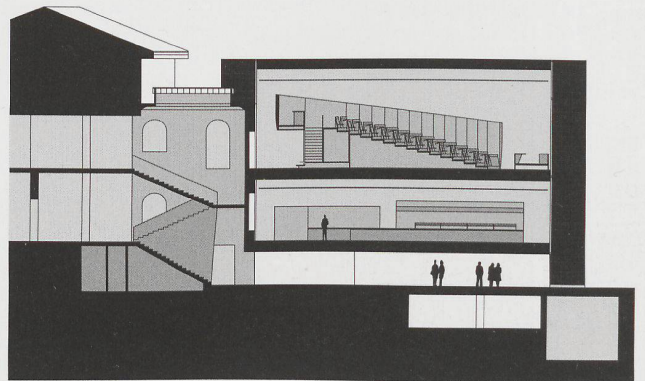
Sezione longitudinale
