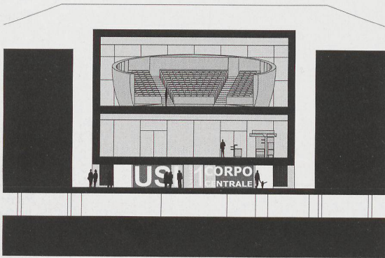
Sezione trasversale
