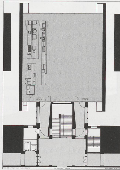
Pianta primo piano
