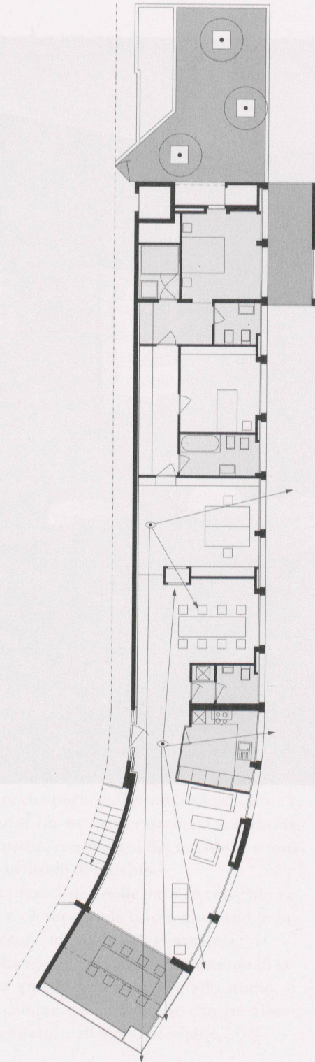
Pianta di progetto
