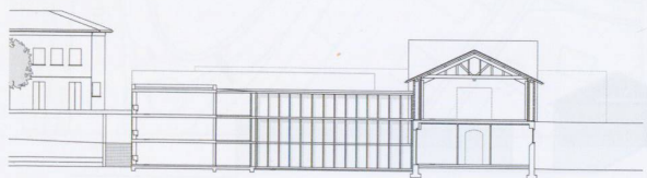
Sezione
