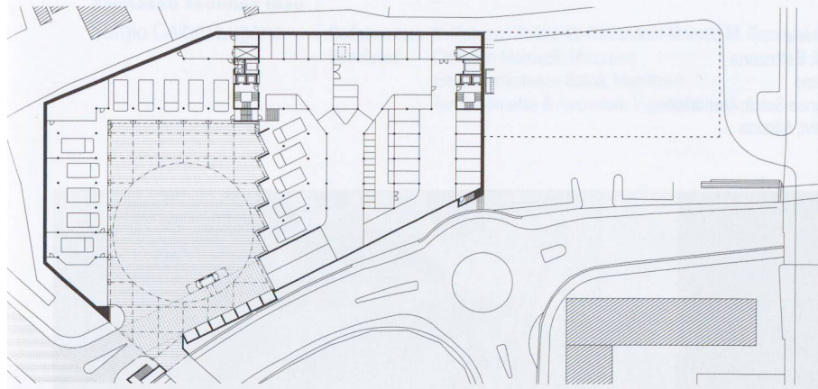
Pianta piano inferiore
