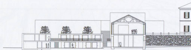
Sezione
