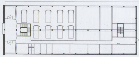
Pianta piano terra
