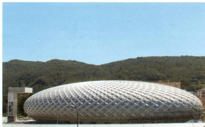
Centro commerciale «Ovale» di Chiasso Architetto: Elio Ostinelli; Chiasso Project Manager: Artech SA, arch. Gianluca Lopes; Lugano Ingegnere guscio: Aurelio Muttoni, Franco Lurati, Miguel Fernandes; Losanna-Mendrisio
