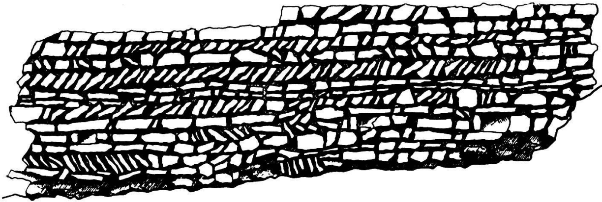
Bild 13. SO-Mauer in Raum XVIII von NO, Strukturzeichnung.
