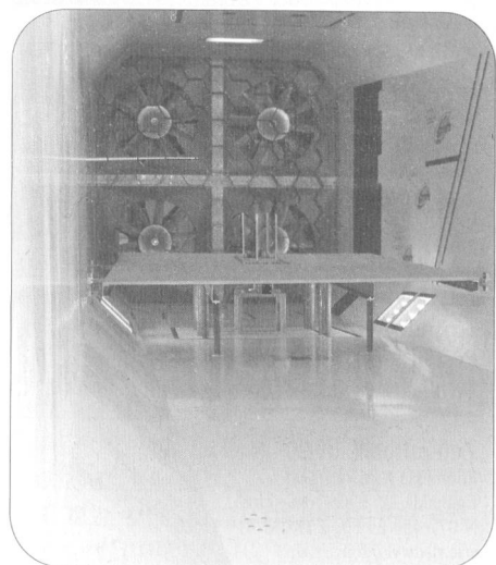
La soufflerie du CMEFE.
