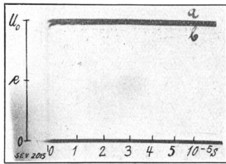
Fig. 4. Umbildung einer Sprungwelle an einer vielspüligen Zylinderwicklung (Scheibenwicklung, 4 Doppelspulen von je 375 Windungen in Reihe). a) Welle am offenen Ende U_0 . b) Klemmenspannung u der Spule.
