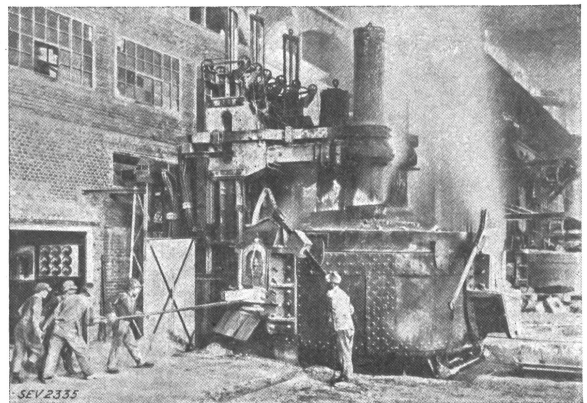
Fig. 18. Elektrischer Stahlschmelzofen des Elektrostahlwerks Aosta; Fassungsvermögen 20 t; hydro-elektrische Hand- und automatische Elektrodenregelung; hydraulische Kippvorrichtung.
