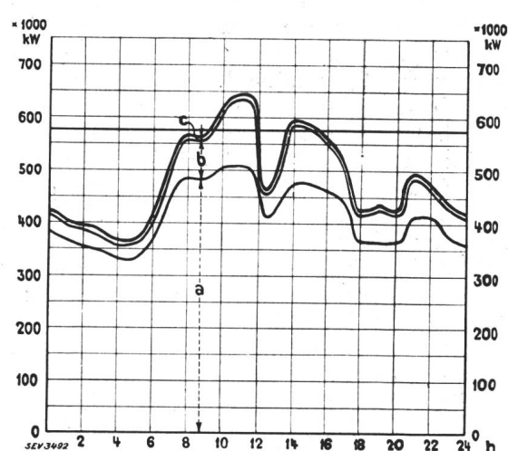
Fig. 9. Répartition de la production le 14 juin 1933. (Capacité de production maximum des usines au fil de l'eau.)
