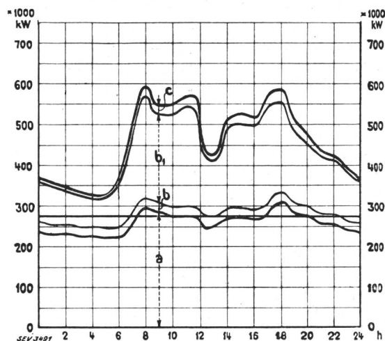
Fig. 8. Répartition de la production le 18 janvier 1933. (Capacité de production minimum des usines au fil de l'eau.)
