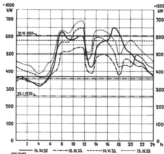
Fig. 6. Graphiques journaliers de la charge totale.
