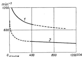
Fig. 2. Leistungen und Drehzahlen von Fahrzeugs-Dieselelektrogruppen. 1 Kleine Gruppen. 2 Grosse Gruppen.
