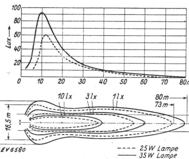
Isoluxkurven auf der Fahrbahn.
