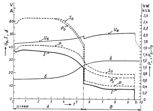
Fig. 6. Betriebsdiagramme einer Ladeperiode von einer Panzerplattenbatterie, 20 Pb-Zellen, max. Strom 38 A, Kapazität 200 Ah. I Ladestrom in A. U_B Ladespannung und Batteriespannung in V. \delta Säuredichte in den Zellen. P_- Gleichstrom-Ladeleistung in kW. P_D Drehstrom-Wirkleistung in kW. S_D Drehstrom-Scheinleistung in kVA. A Hauptladung: 192 Ah. B Nachladung: 36 Ah.
