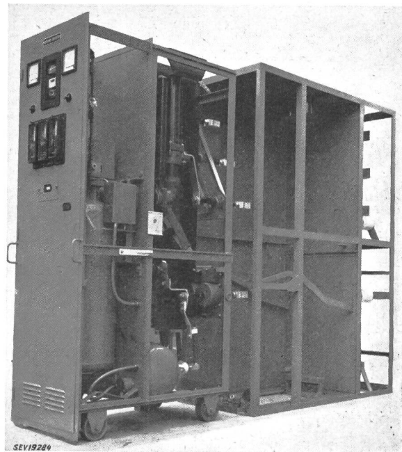
Fig. 2 Ansicht des Feldes Fig. 1, Apparatwagen vollständig ausgezogen
