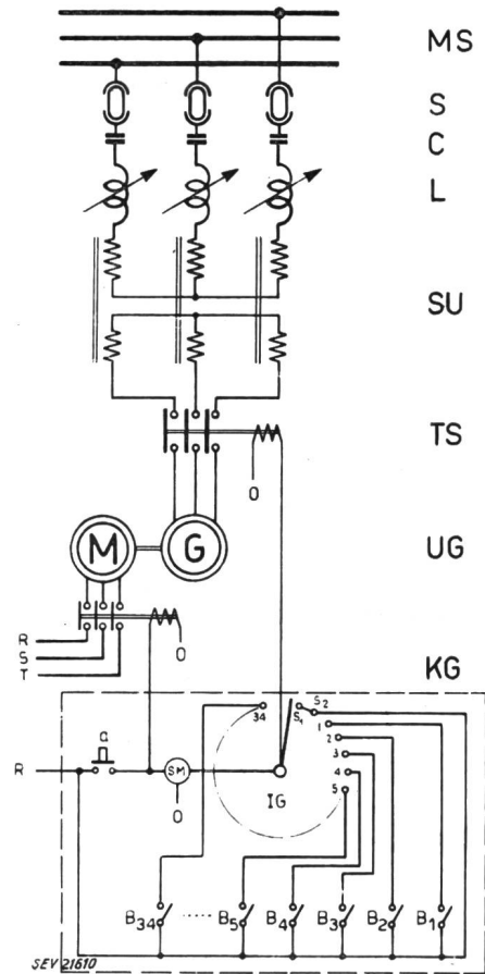
Fig. 10 Prinzipschema einer Sendeanlage (System Ghielmetti)
