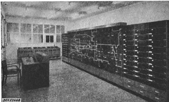
Fig. 2 Vorderansicht der Netzmodellanlage mit Messtisch, Generatorpulten, Knotenpunkttafel und seitlichen Fächerschränken
