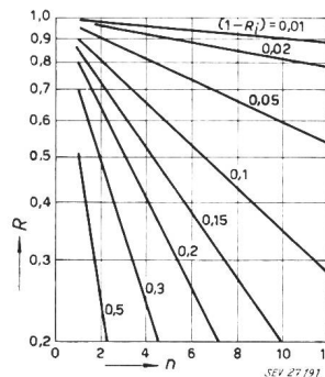
Fig. 1 Funktion der Zuverlässigkeit R Zuverlässigkeit einer ganzen Schaltung; n Anzahl Bauelemente in der Schaltung; R_i Zuverlässigkeit der einzelnen Bauelemente; (1 - R_i) Unzuverlässigkeit der einzelnen Bauelemente
