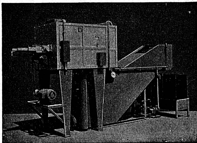
Four continu, à moufle, type 10 MVi 20, pour la trempe blanche et la carbonituration.
