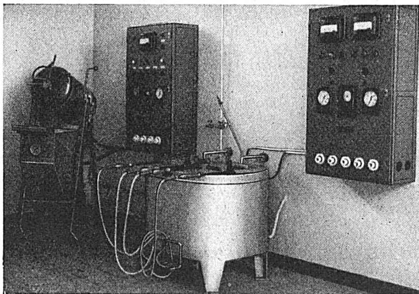
Installation de trempe et revenu blanc de petites pièces d'horlogerie
