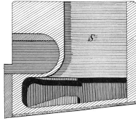
Gewehr (Schloss gespannt). 1/3 nat. Grösse.
