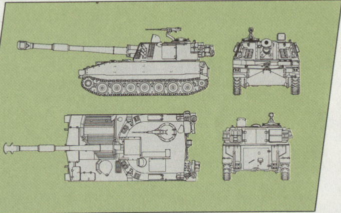
CH Panzerhaubitze M-109
