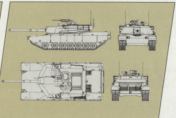
NATO Kampfpanzer ABRAMS
