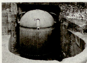
5,3-cm-Fahrpanzerkanone 1887
