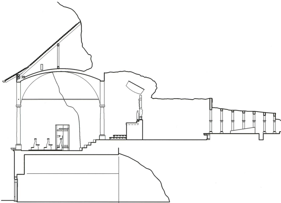
Abb. 7 Längsschnitt durch die Verena- kapelle mit angebaute Vor- halle und nach hinten natür- liche und künstliche Höhle mit dem Kreuzaltar und dem Heiliggrab. Planaufnahme 1:100, wwB Architekten, Februar 2019.
