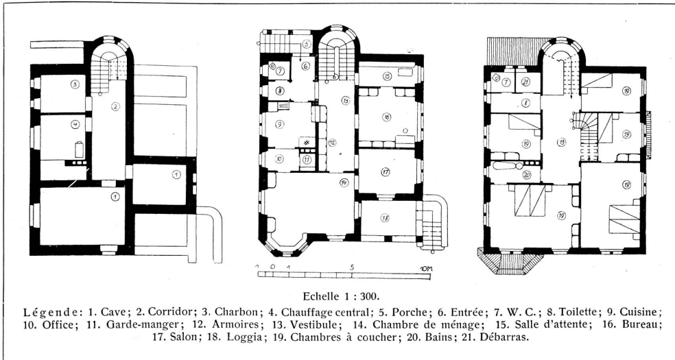
Maison d'habitation du D r O. Kubli à Glaris. — Vue perspective et plans. Architecte: Fr. Glor-Knobel, Glaris.
