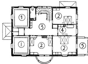
Plans de la Villa Eymann à Langenthal. — Architecte : O. Honegger, Zurich. — Echelle 1 : 400.
