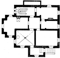
Villa Naef à Küsnacht (Zurich). — Plans 1 : 400. — Architecte : O. Honegger, Zurich.
