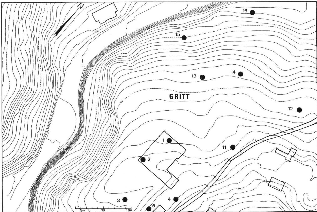
Bild 2. Situation der Ueberbauung mit Lokalisierung der Bohrungen 1973 (Bohrung 5 zirka 15 m weiter unten). Abstand der Höhenkurven 1 m. Aufnahme: Ingenieurbureau Holinger AG, Eintragungen: Dr. W. Mohler. Das Altersheim Gritt im Bereich der Bohrungen 1 und 2.
