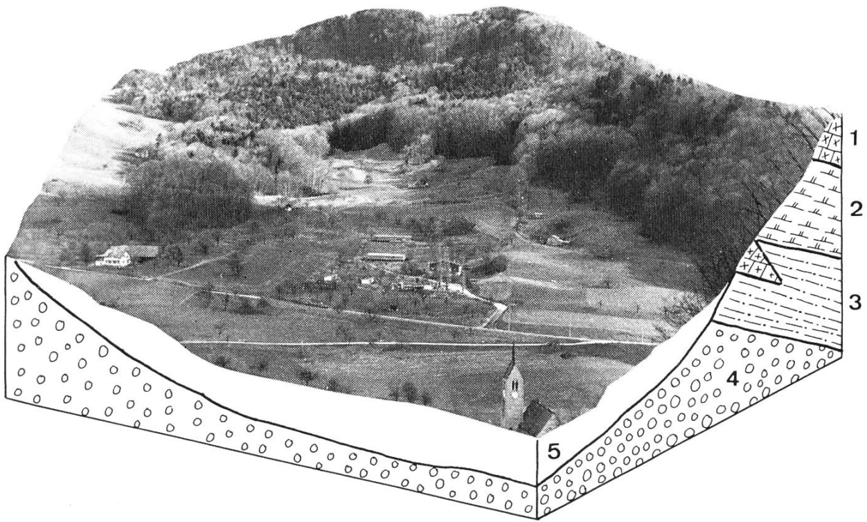
Bild 3. Bergrutschgebiet Dielenberg, gesehen von Westen. Photo und Blockdiagramm von Dr. Peter Suter, geologische Profile nach Dr. Lukas Hauber. 1 Hauptmuschelkalk, 2 Anhydritgruppe, 3 Keuper, 4 Juranagelfluh (Tortonien), 5 Bergrutschmaterial.
