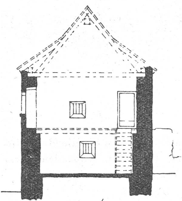
QUER - SCHNITT
