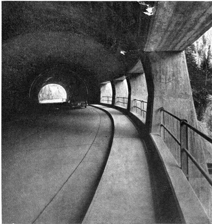
Lukmanierpaß-Straße, Betonbelag in Galerie
