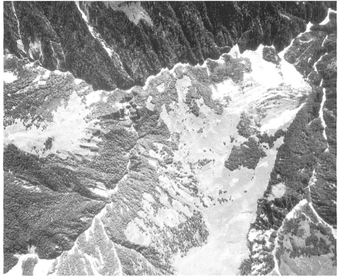
Schuderser Rutschgebiet 1970. (Quelle: ELT 1971)
