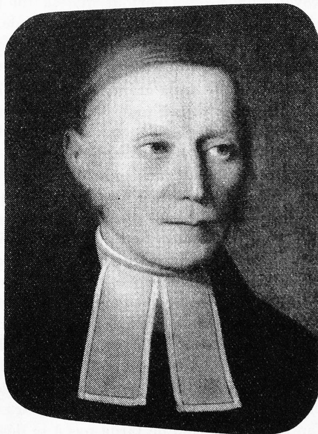
Theodor Fliedner (1799—1864)
