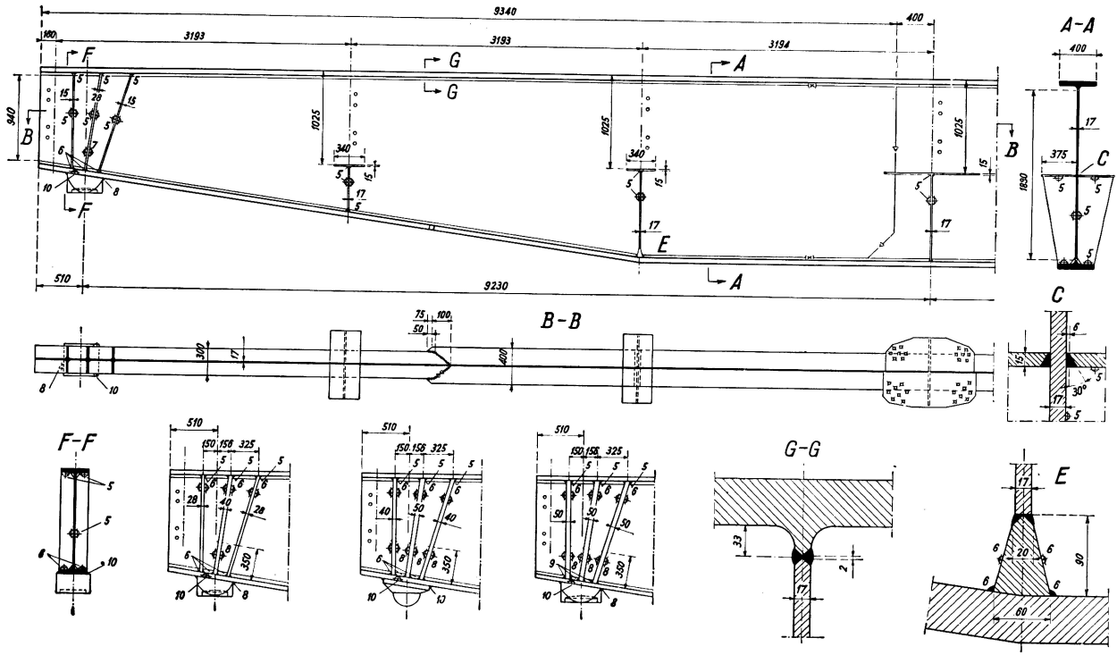
Fig. 11. Pont de Pålssund. Entretroises.
