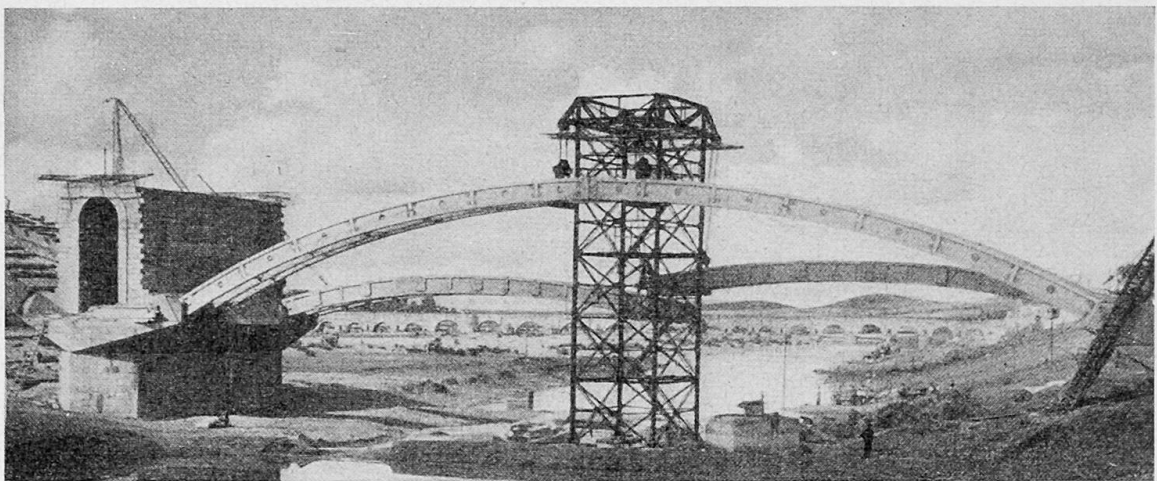
Fig. 12 - Pont de Merida sur le Guadiana - Montage des anneaux auto-cintrés.
