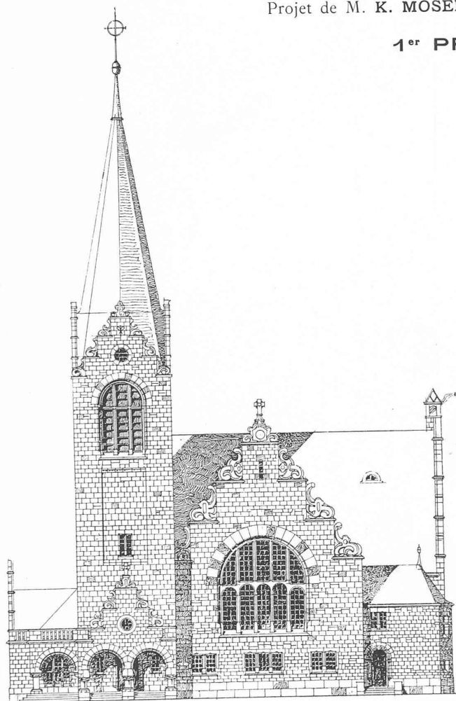
FAÇADE DU COTÉ DE LA FELLENBERGSTRASSE (1 : 400)
