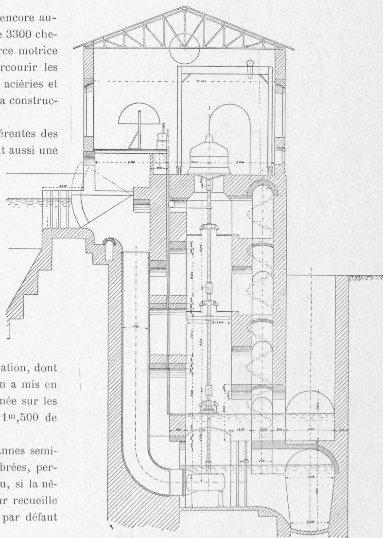
Fig. 4. — Usine centrale de Papigno. — Coupe transversale.
