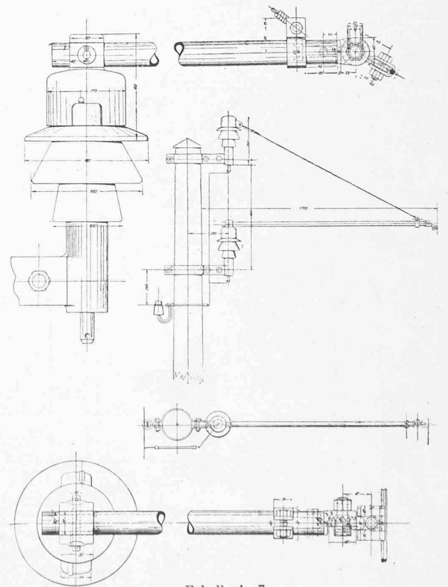
Echelle 1 : 7.
