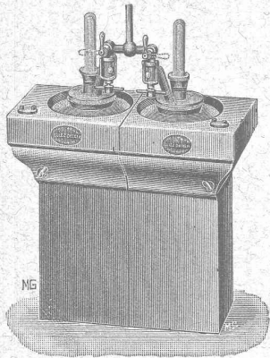
Appareil accouplé complet. Cet appareil se charge par des briquettes de carbure comprimé, il est destiné à l'éclairage des voitures de chemin de fer, fourgons, locomotives, etc., ainsi qu'à différents locaux.
