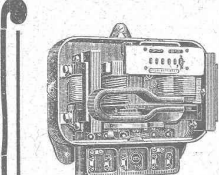
Compteur pour courant alternatif triphasé.
