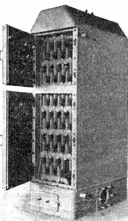
Calorifère récupérateur breveté
