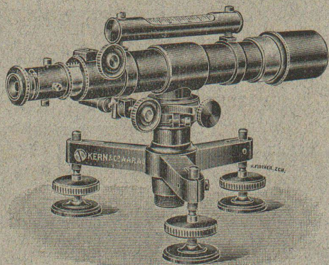
Niveau à lunette N° 102
