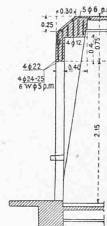
Fig. 20. Couvertes 918-919. 1 : 80.
