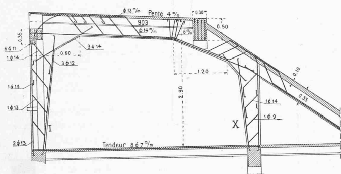
Fig. 19. — Vue du sommier 903 et des piliers I-X. — 1 : 80.
