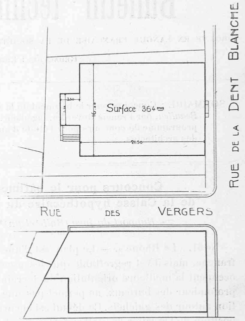
Plan de situation. — 1 : 600.
