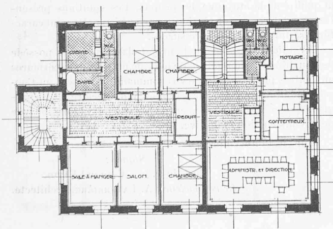
Plan du premier étage. — 1 : 300.
