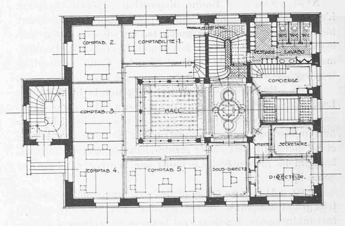
Plan du rez-de-chaussée. — 1 : 300.
