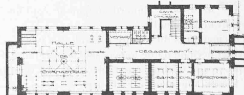
Plan du sous-sol - 1 : 800
